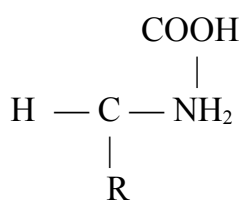
D-Amino acid
