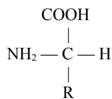
L-Amino acid
